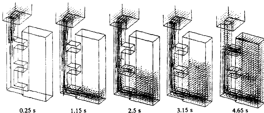
图 3 阶梯式浇注系统充型流动过程数值模拟结果 (速度矢量法)
