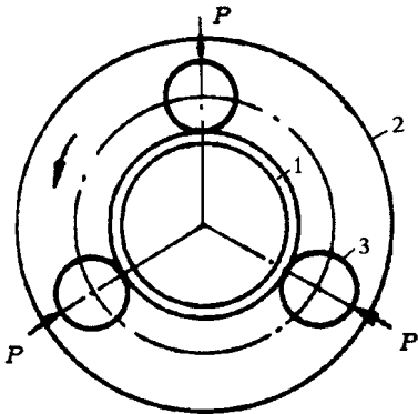
图 1 滚切机工作示意图
