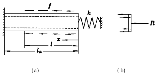
图 1 温度变化引起的管道变形伸长
