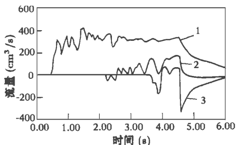
图 4 各层内浇道流量随时间的变化 (计算结果)
